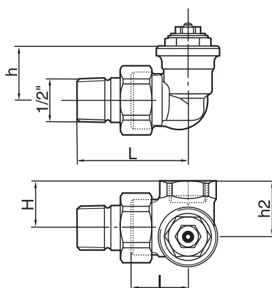
Abb. 9. Winkeleck
