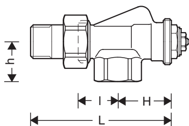
Abb. 8. Axial
