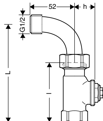
Abb. 10. Durchgang mit Bogentülle
