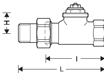
Abb. 7. Durchgang
