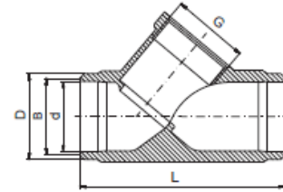
Anschweißenden DIN 3239 "A" / welded connection DIN 3239 "A"
