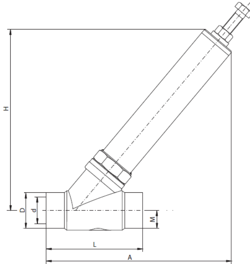
Anschweißenden DIN 11850-2 "M" / welded connection DIN 11850-2 "M"
