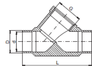
Anschweißenden DIN 11850-2 "M" / welded connection DIN 11850-2 "M"
