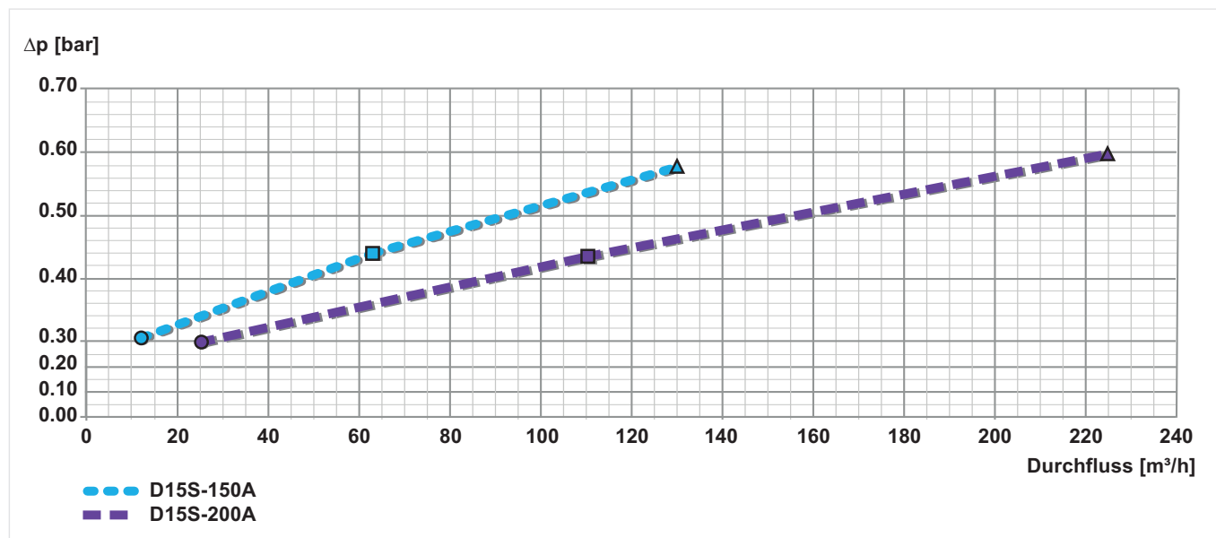
Abb. 3 Druckabfall innerhalb des Ventils ist abhängig vom Durchfluss und der verwendeten Anschlussgröße (Größen 150-200)
