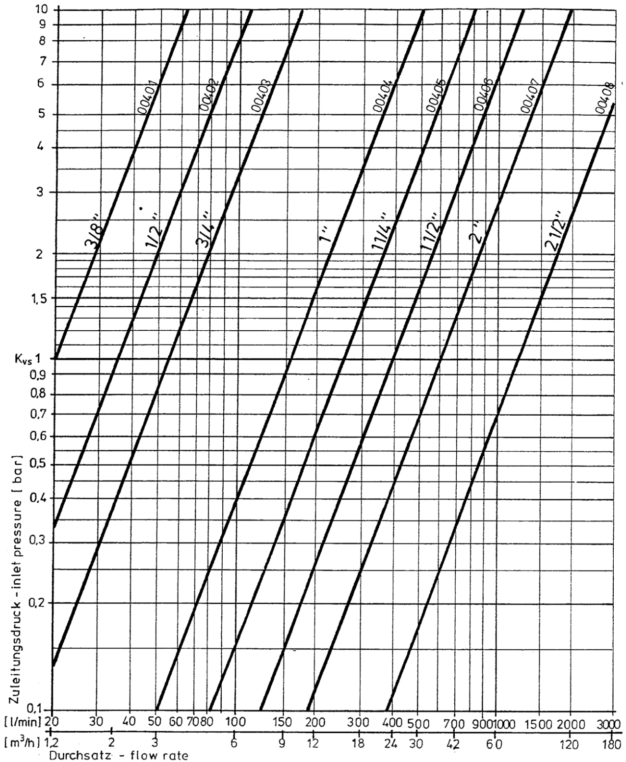
Leistungsdiagramm Performance diagram
