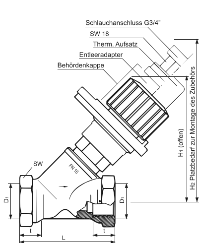
Abb.2 Alwa-Kombi-4 mit Innengewinde
