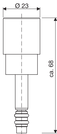
Abb.4 Thermischer Regelaufsatz für Alwa Kombi-4
