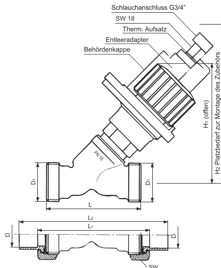
Abb.3 Alwa-Kombi-4 mit Außengewinde
