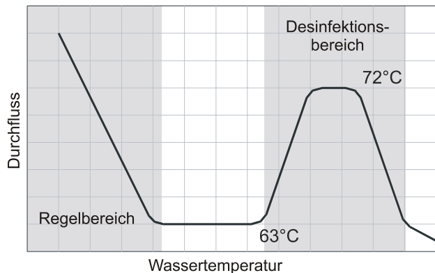
Abb.1 Beziehung zwischen Durchflussrate und Wassertemperatur
